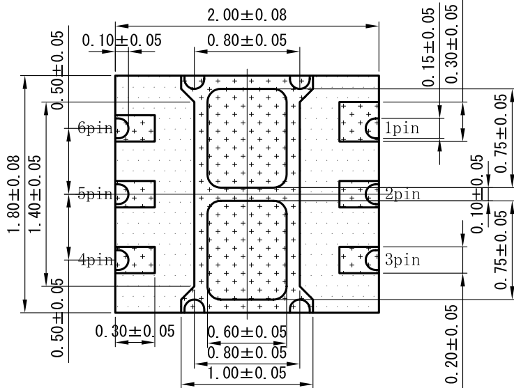
実装面
