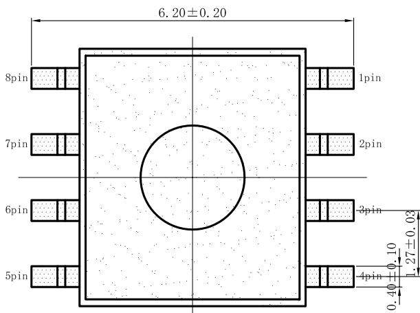
実装図
