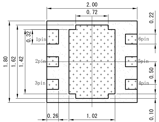
インナーリード部図
