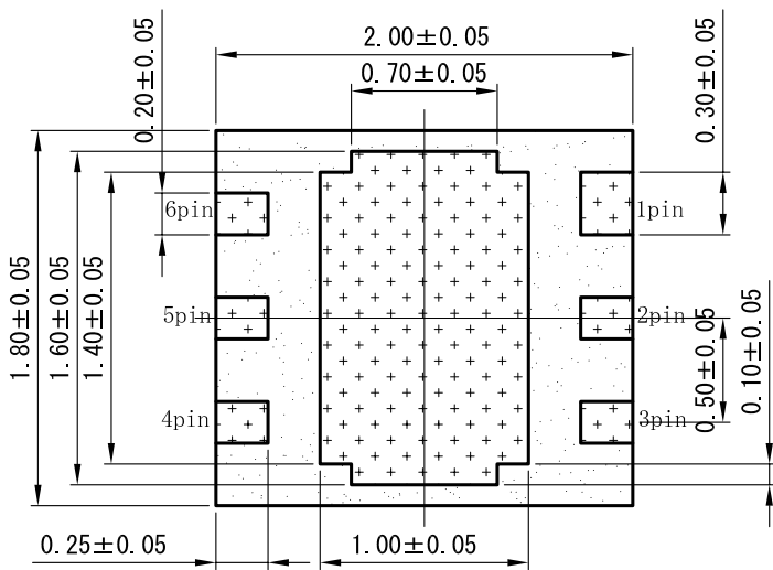
実装面
