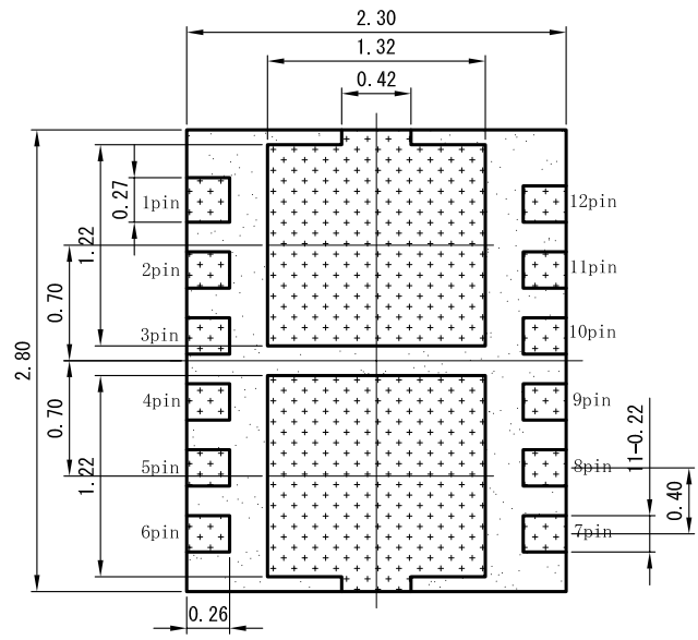
インナーリード部図
